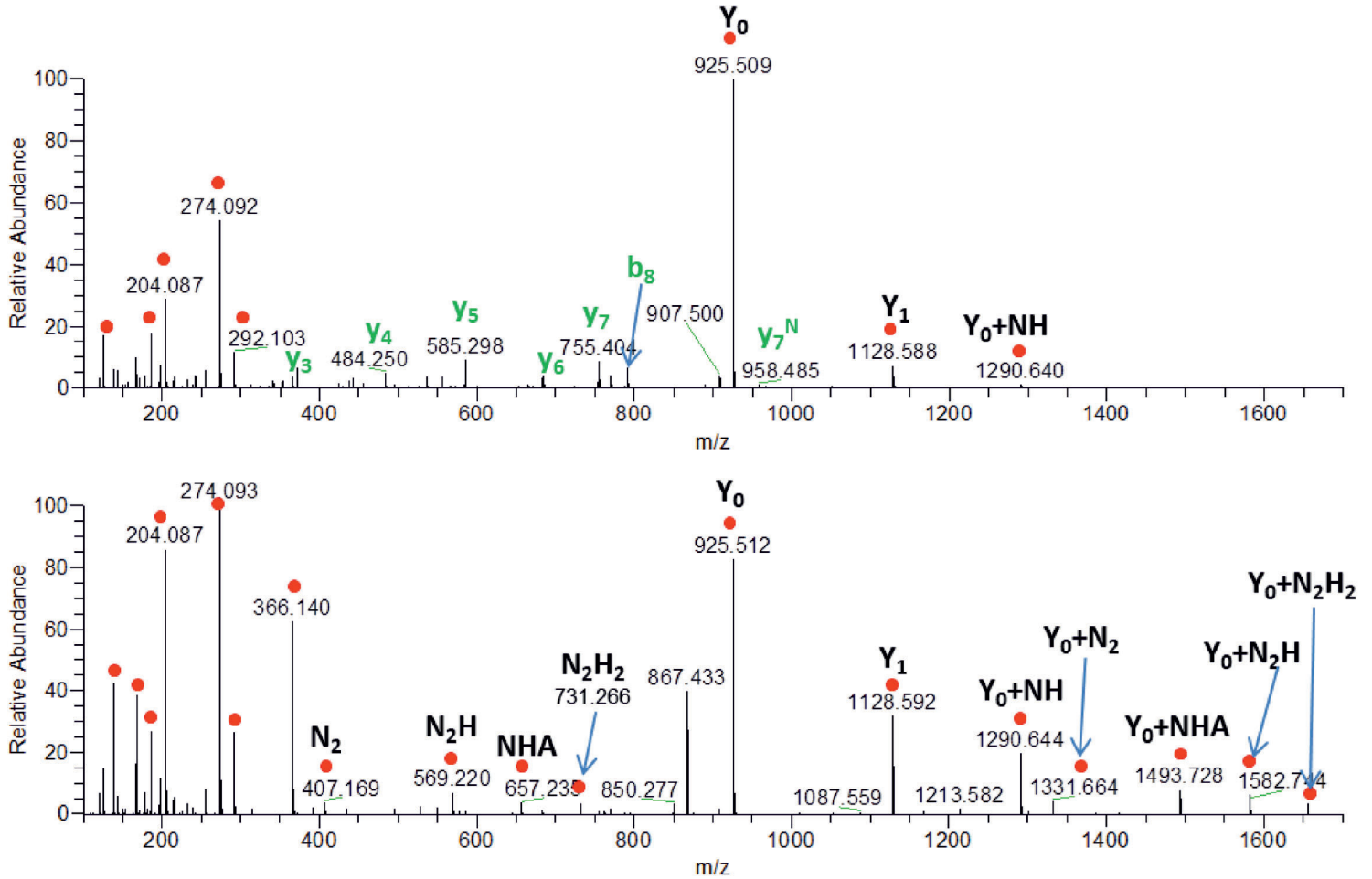
12.4. ábra. Az AVAVTLQSH peptid két glikoformájáról felvett HCD spektrum. A peptid-fragmentációból származó ionokat zölddel, a glikán-fragmentációból származókat pirossal jeleztük. A nagyobb glikánt hordozó O -glikopeptid HCD spektrumában már nem figyelhetők meg peptid fragmens ionok.
